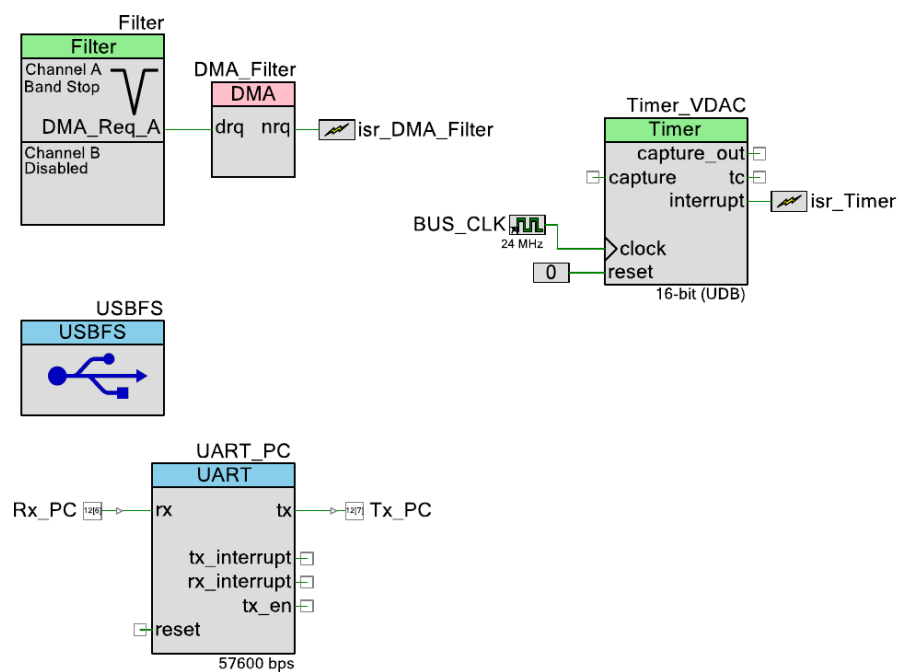
Figura 7: Hito 03, Comparison , hoja digital: filtro y DMA, temporizador de 16 bits alimentado por el reloj de bus, USBFS y UART a 57600 bit/s. Esta hoja completa la arquitectura visible en la figura anterior y registra las alternativas de temporización y comunicación disponibles en el banco.
