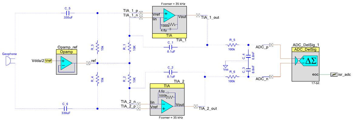
Figura 4: Hito 02, Tesis, hoja analógica: el acondicionamiento pasa a dos ramas TIA, polarizadas alrededor de V_{DDA}/2 , y termina en un ADC \Delta\Sigma de 17 bits. Los capacitores de realimentación y las redes RC anteriores al ADC introducen una conformación espectral explícita que no existía en la revisión inicial.
