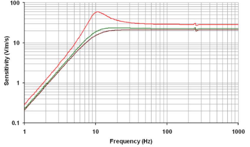
Figura 1: El transductor disponible y su respuesta publicada. A la izquierda se muestra un SM-24 montado en carcasa con punta de acoplamiento [Jagadesh, 2012]; a la derecha, las curvas de sensibilidad del folleto del fabricante para distintas condiciones de amortiguamiento [Sensor Nederland B.V., 2006]. La imagen permite separar dos conceptos que luego se modelan matemáticamente: el montaje mecánico del receptor y la dinámica del elemento interno.
